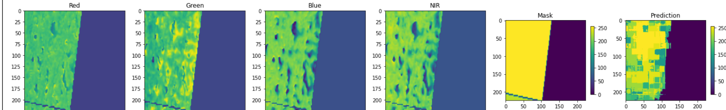
Resultado modelo segmentación semántica: Clorofila
