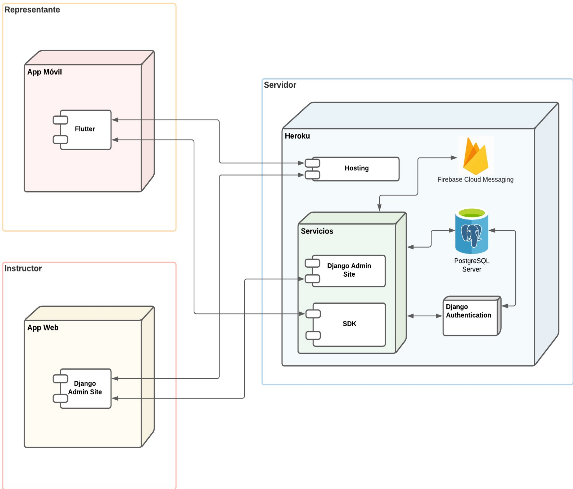
Figura 4. Diagrama de despliegue de la solución EFConecta
